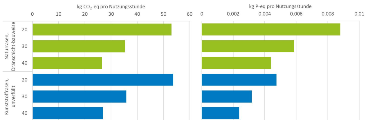
Abbildung 14: Treibhausgasemissionen in kg CO 2 -eq (links) und Süsswasser-Eutrophierung in kg P-eq (rechts) pro theoretische Nutzungsstunde (800 h für Naturrasen mit Dränschicht und 1600 h für unverfüllten Kunststoffrasen) in Abhängigkeit zur Lebensdauer. Je länger die Lebensdauer, desto kleiner sind die Umweltauswirkungen pro Nutzungsstunde.
